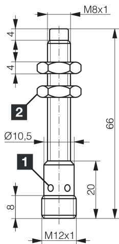
1) LED 4 x 90° (gelb) 2) Schlüsselweite 13 mm BK: schwarz BN: braun BU: blau
