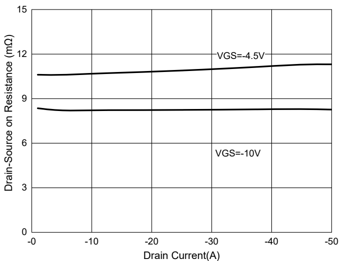
Fig. 5 - R_{DS(ON)} - I_D
