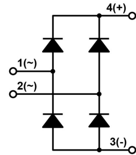
Rectifier Bridge
