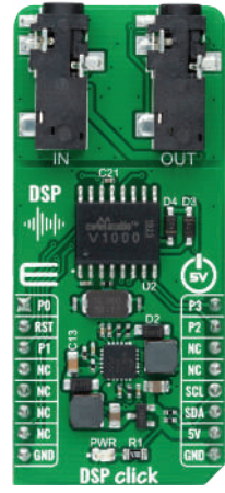
DSP Click
