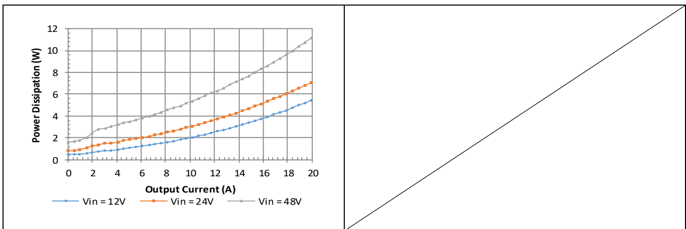
Vo = 3.3 V
