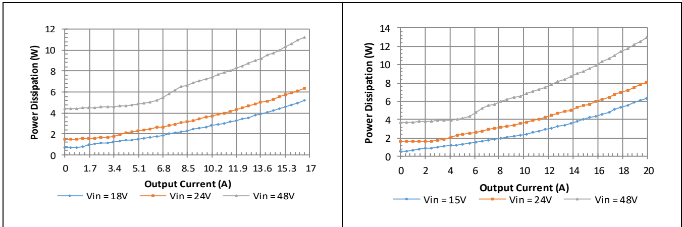
Vo = 15 V
