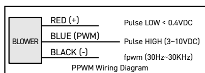
PPWM-pos-slope 2008/7/15
