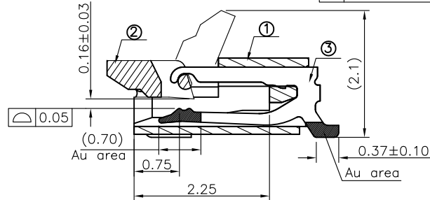
SECTION A-A;SCALE 2:1
